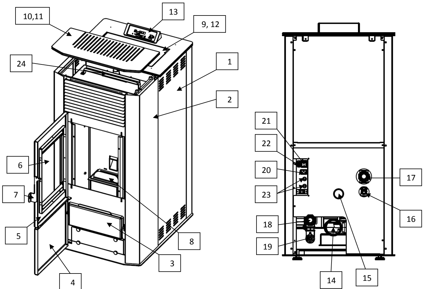
Slika 2 Osnovni delovi peći
